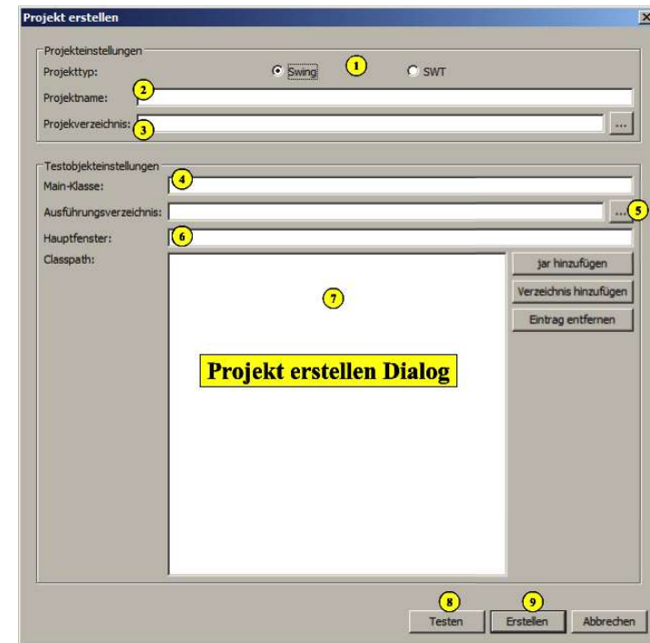
Abbildung 2.2 Projekt erstellen Dialog
