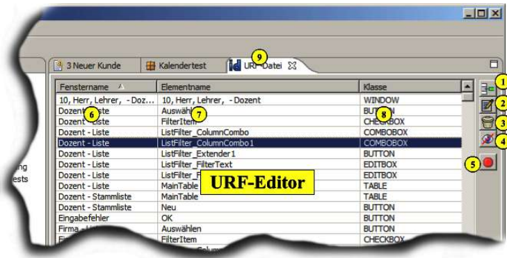
Abbildung 2.5 URF-Editor
