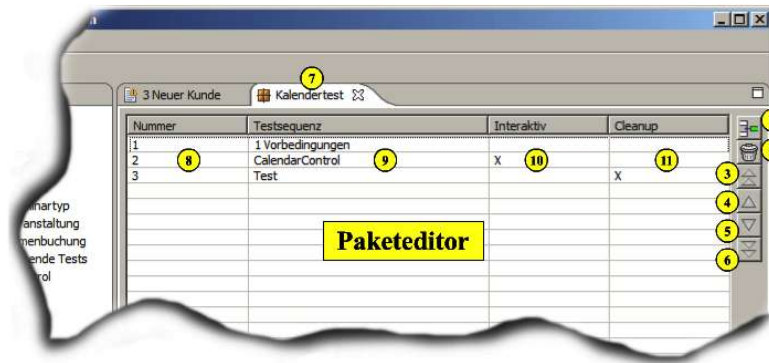
Abbildung 2.4 Paketeditor
