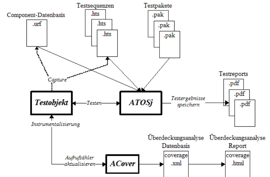
Abbildung 1.1 Testkomponenten und Dateien
