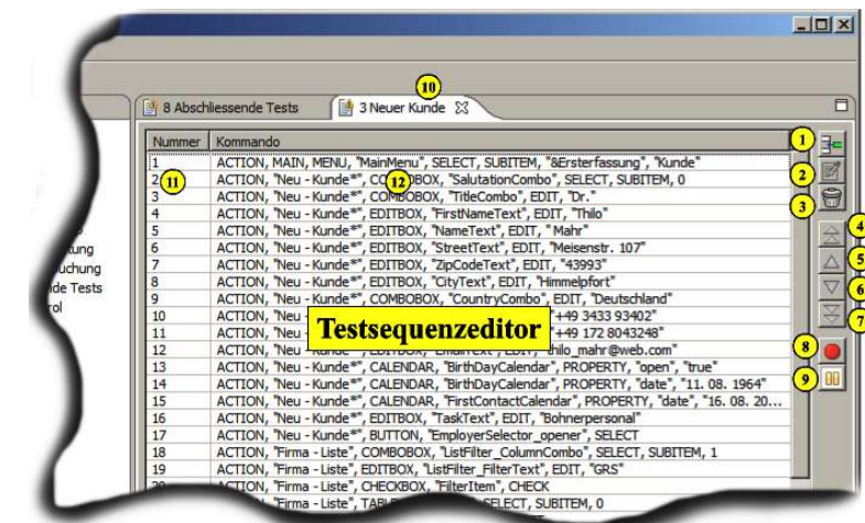
Abbildung 2.3 Testsequenzeditor
