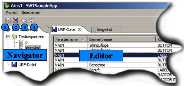
Abbildung 2.1 ATOSj Hauptfenster
