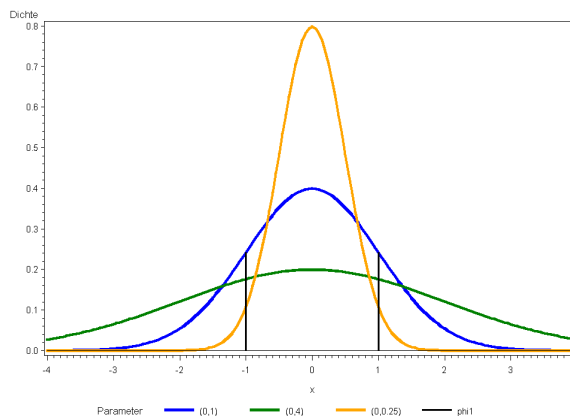
Dichtefunktion verschiedener Normalverteilungen
