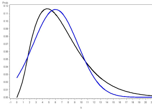
Verteilung der Summe von Quadraten von Zufallsgrößen Xi standardnormal, n=20
