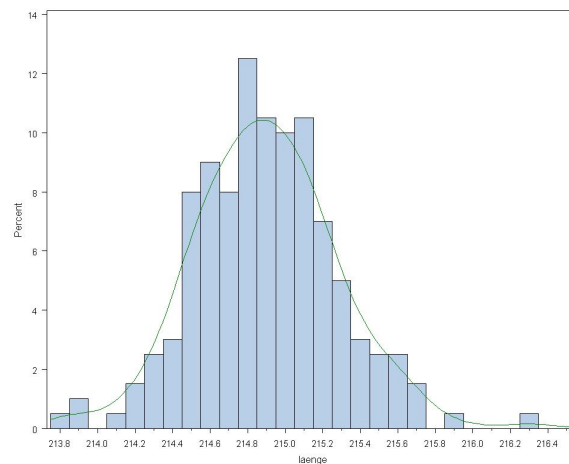
\Delta_0 klein
