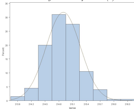
\Delta_0 groß
