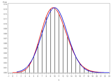
Binomialverteilung-Verteilung B(100,0.1)
