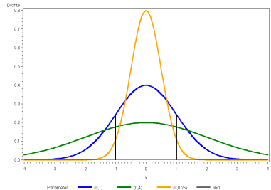
Dichtefunktion verschiedener Normalverteilungen Skalenunterschied
