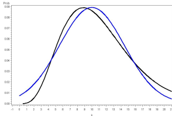
Verteilung der Summe von Quadraten von Zufallsgrößen X1 standardnormal, n=10
