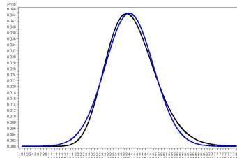
Verteilung der Summe von Quadraten von Zufallsgrößen X1 standardnormal, n=40
