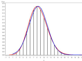
Binomialverteilung-Verteilung B(50, 1/6)
