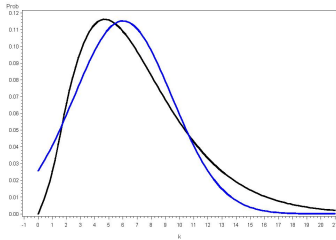
Verteilung der Summe von Quadraten von Zufallsgrößen X1 standardnormal, n=10
