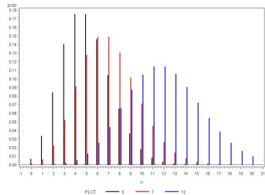
Poisson-Verteilung mit \lambda=5, 7, 12
