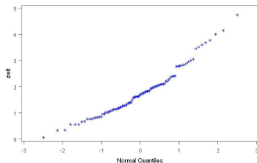
Lebensdauer von Kühlaggregaten (in Jahren)
