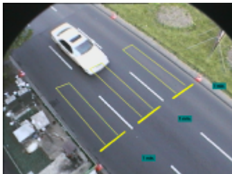
Abb.1: Erfassungsbereich der Kamera und Konfiguration von Autoscope Solo mit Geschwindigkeitsdetektoren (gelbe Vierecke) und Zähl-detektoren (gelbe Balken)
